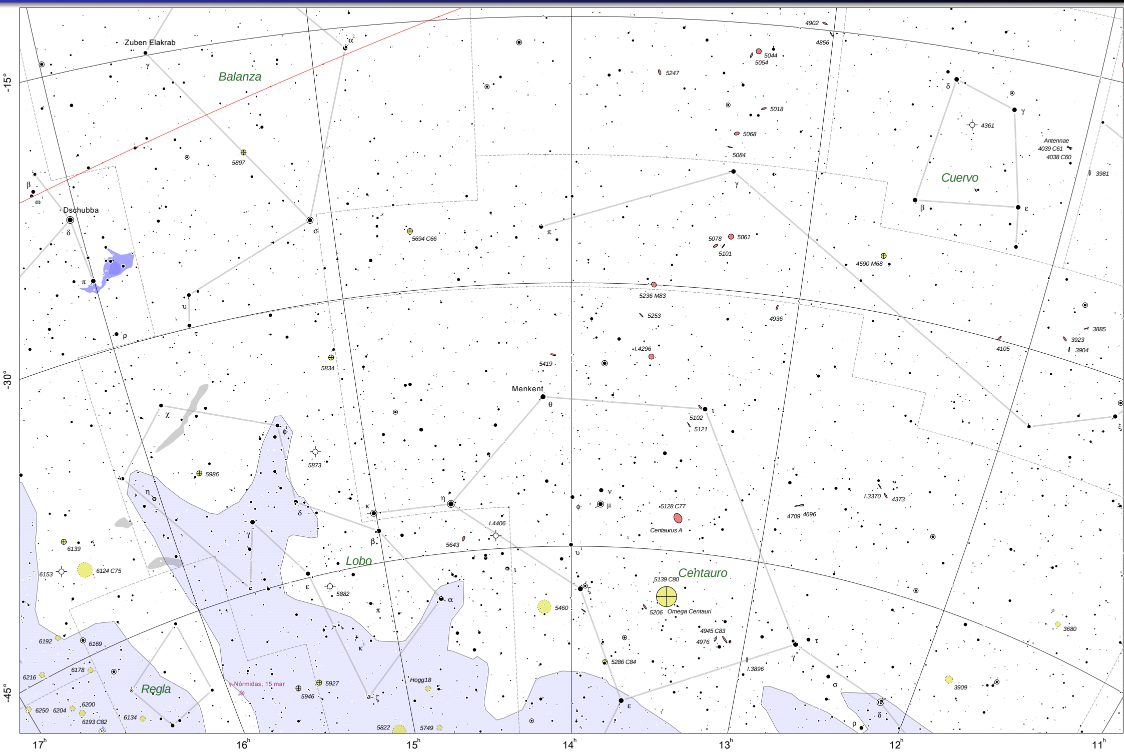
Carta 21, 30° alrededor de 14.0h, -35.0° (Centauro, Hidra, Lobo, Balanza)
