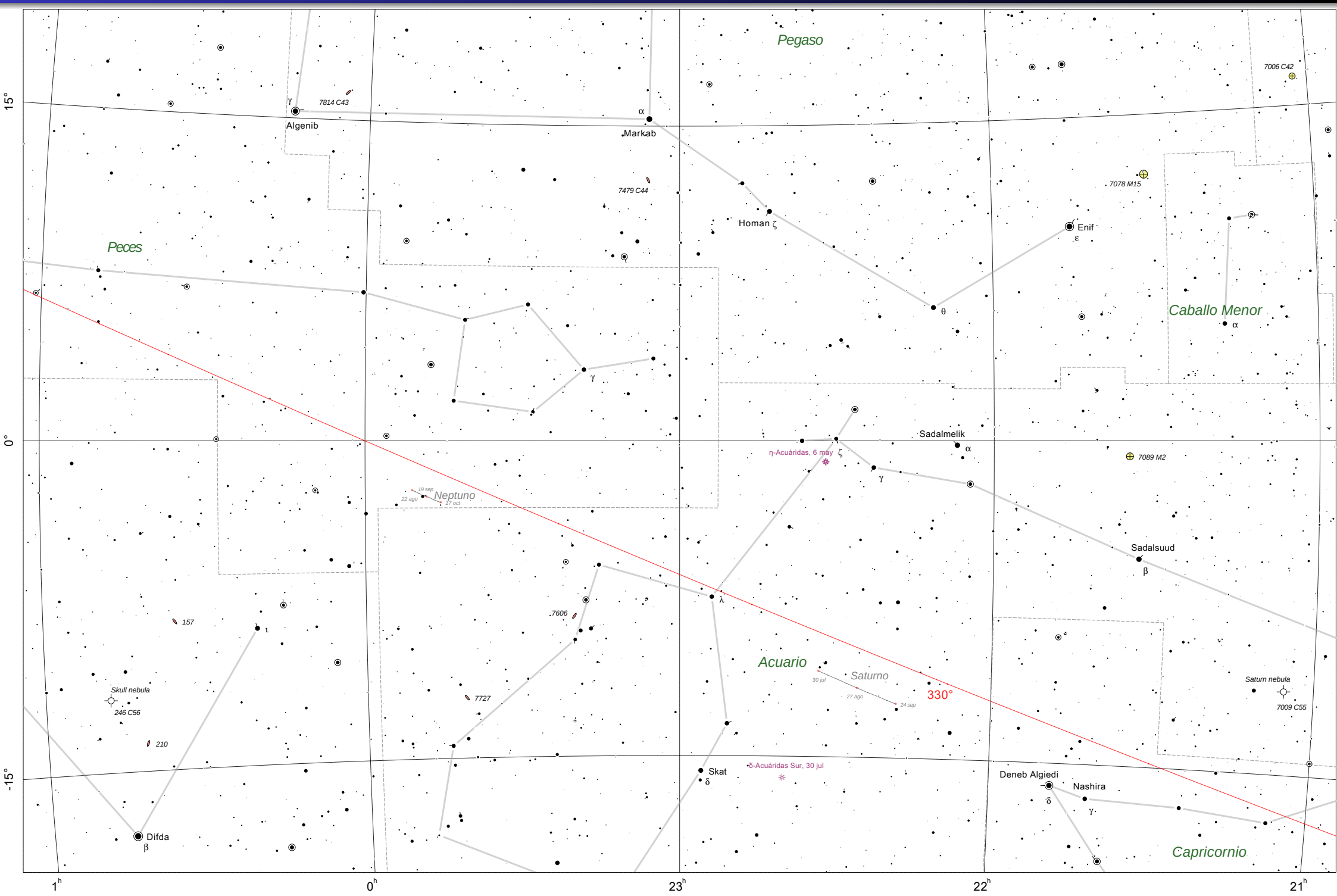
Carta 17, 30º alrededor de 23.0h, 0.0º (Peces, Pegaso, Acuario, Ballena)
