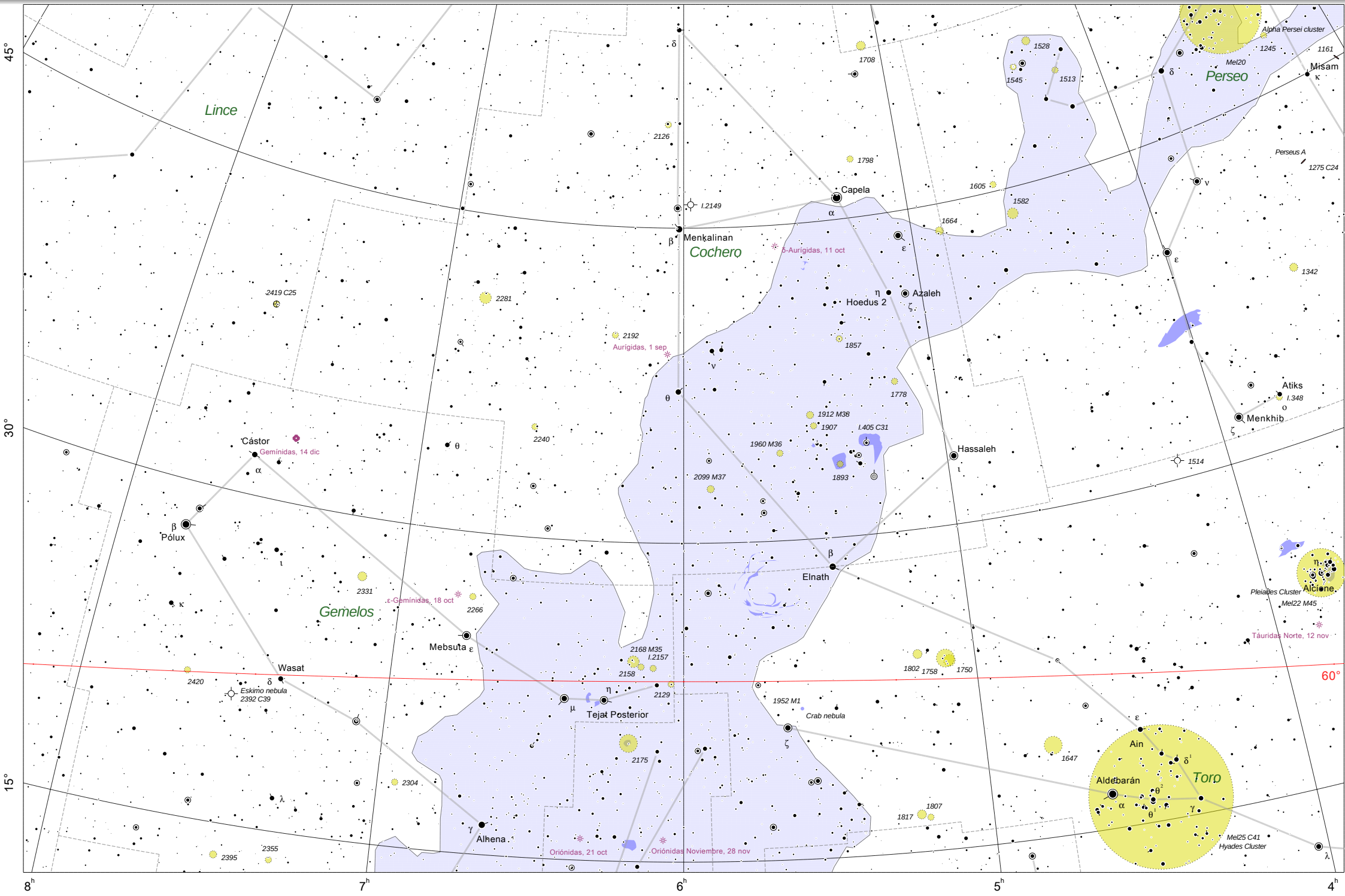
Carta 5, 30º alrededor de 6.0h, 35.0º (Cochero, Gemelos, Toro, Orión)
