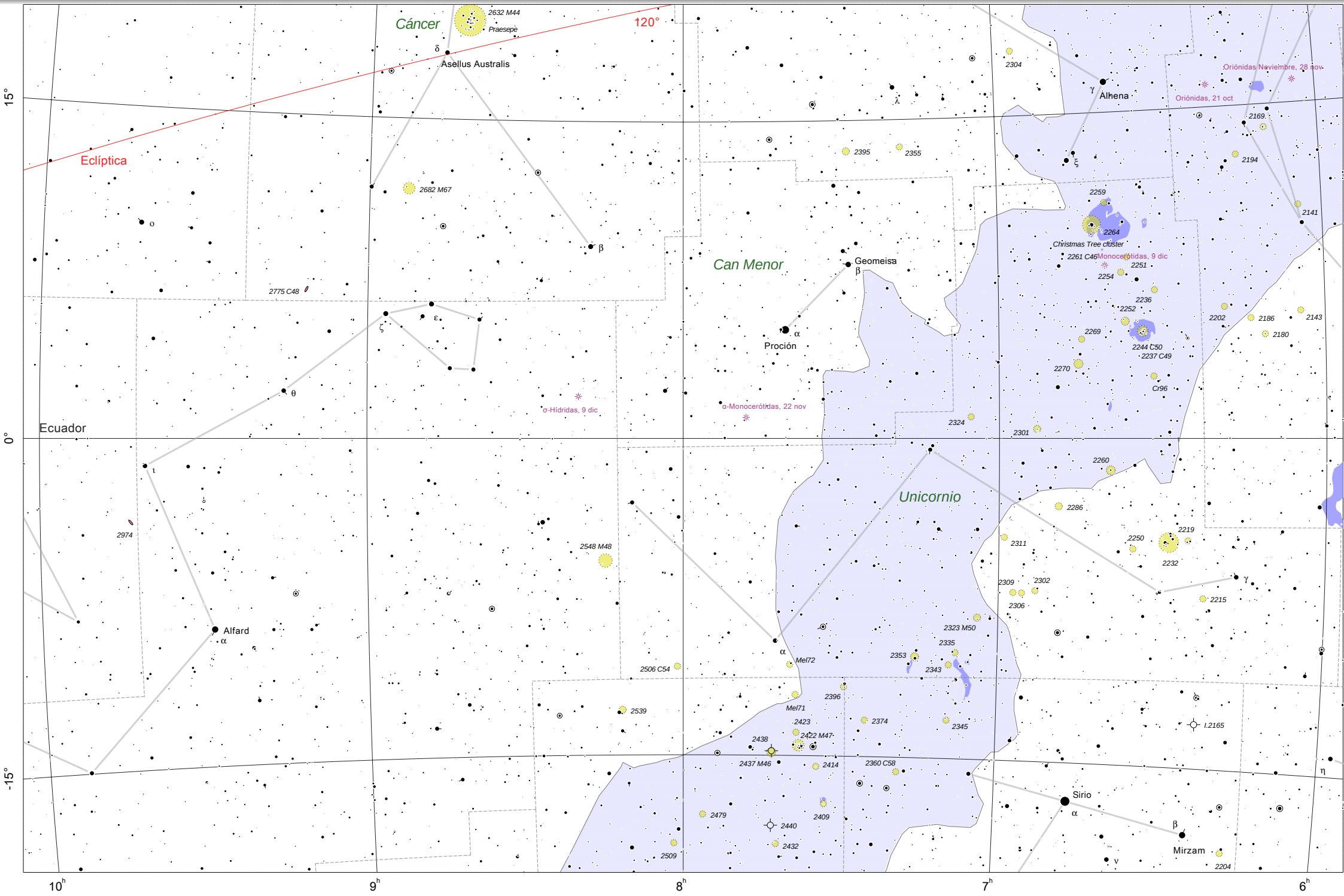
Carta 12, 30º alrededor de 8.0h, 0.0º (Can Menor, Hidra, Unicornio, Cáncer)
