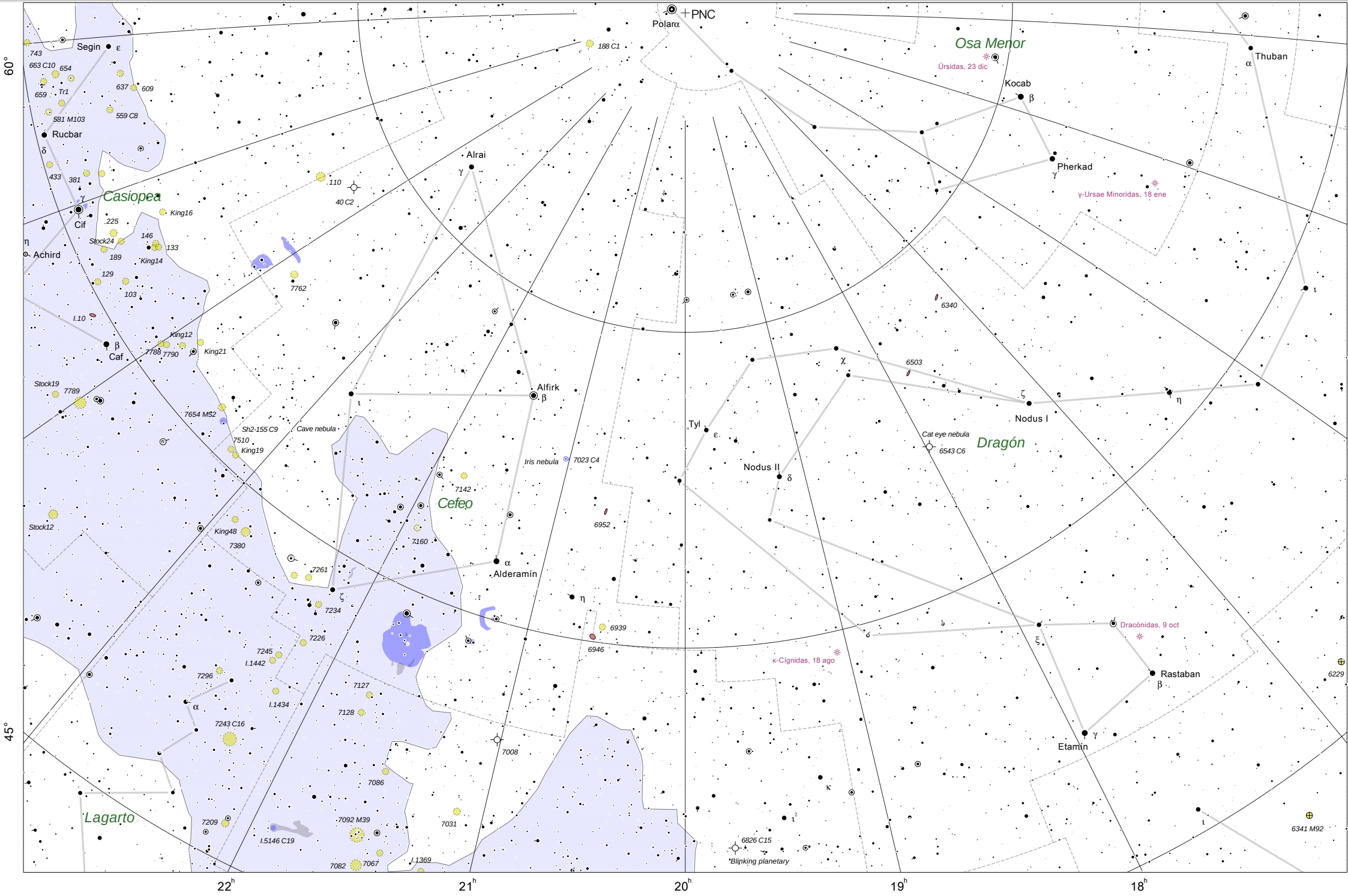
Carta 3, 30º alrededor de 20.0h, 70.0º (Dragón, Cefeo, Cisne, Casiopea)
