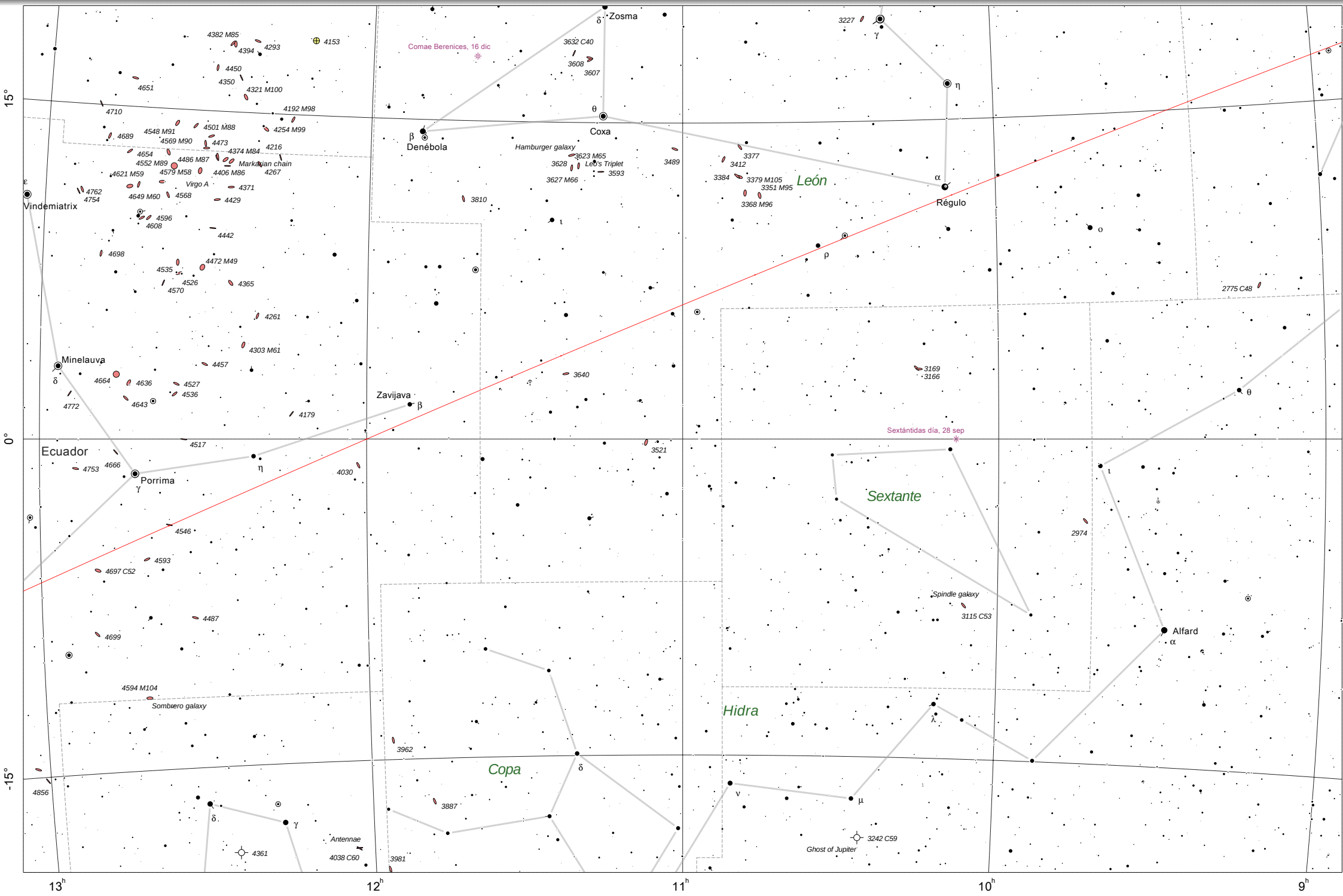
Carta 13, 30º alrededor de 11.0h, 0.0º (León, Sextante, Virgen, Copa)
