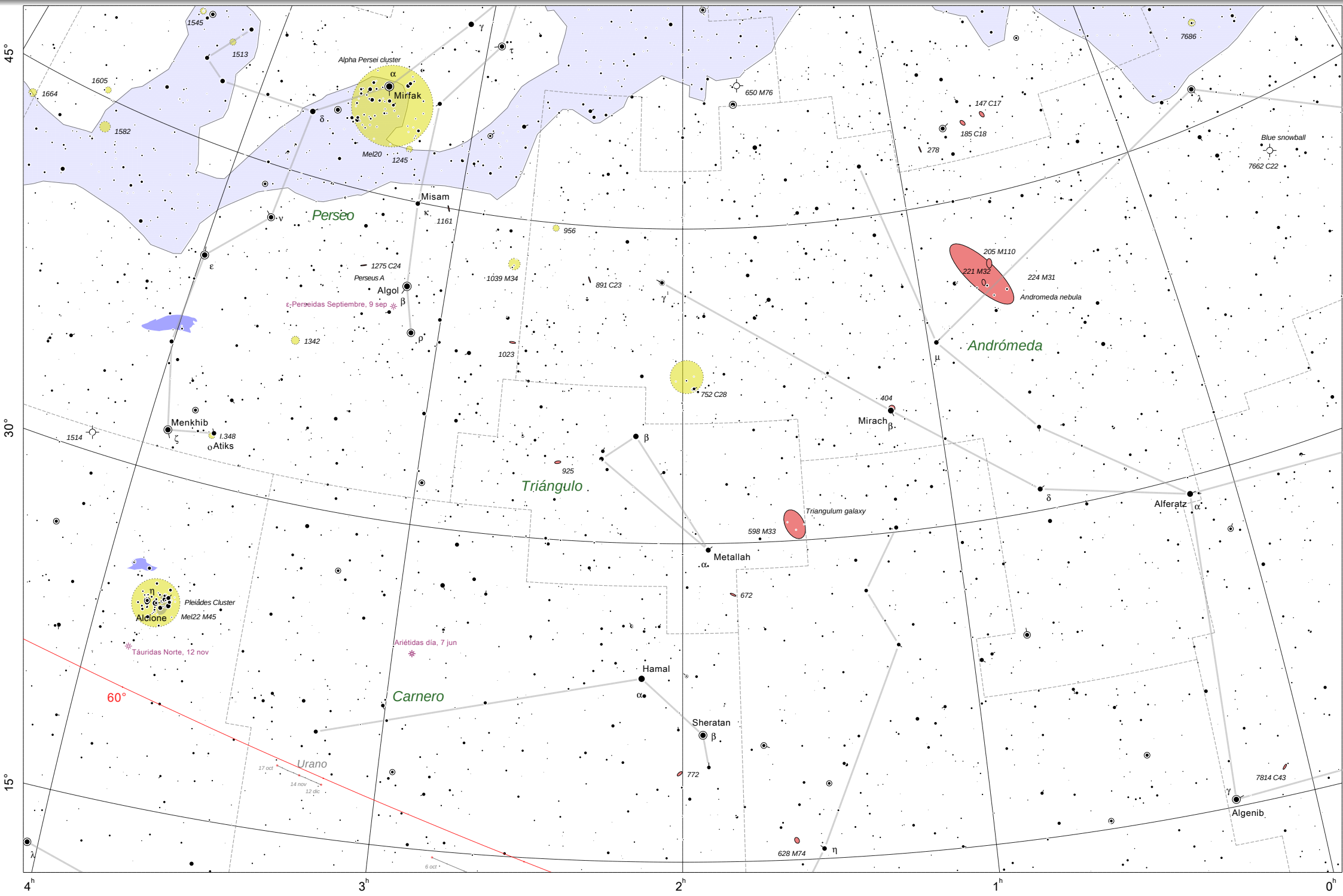
Carta 4, 30º alrededor de 2.0h, 35.0º (Triángulo, Andrómeda, Perseo, Peces)
