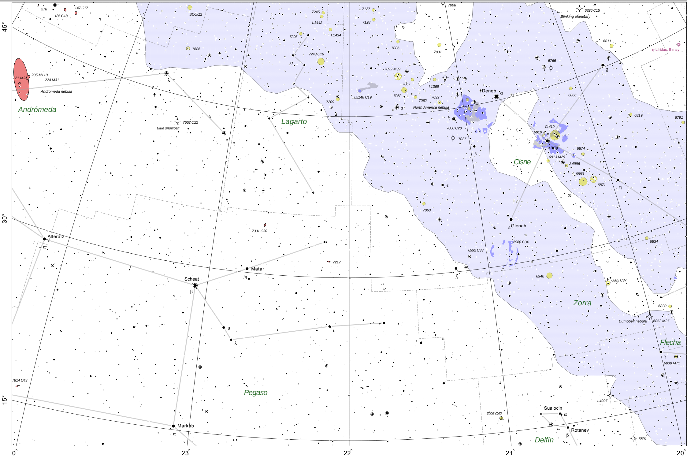
Carta 9, 30º alrededor de 22.0h, 35.0º (Pegaso, Lagarto, Cisne, Zorra)
