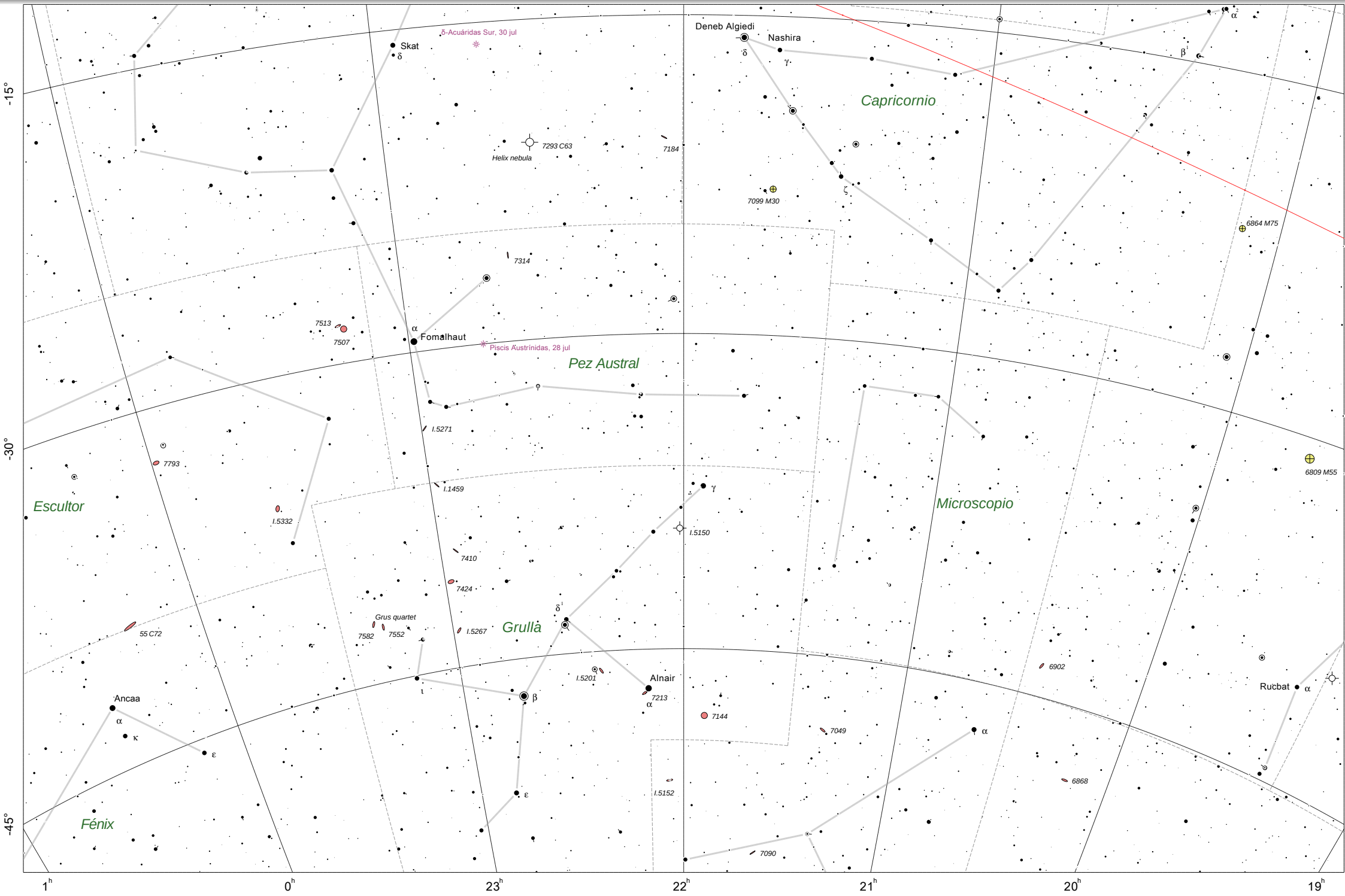
Carta 23, 30° alrededor de 22.0h, -35.0° (Pez Austral, Grulla, Escultor, Acuario)
