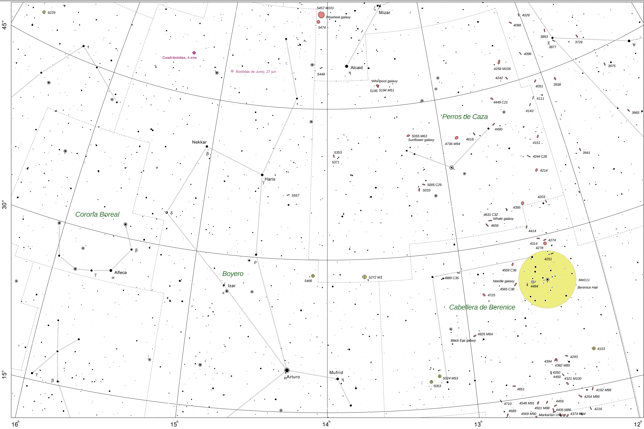
Carta 7, 30º alrededor de 14.0h, 35.0º (Perros de caza, Boyero, Osa Mayor, Cabellera de Berenice)
