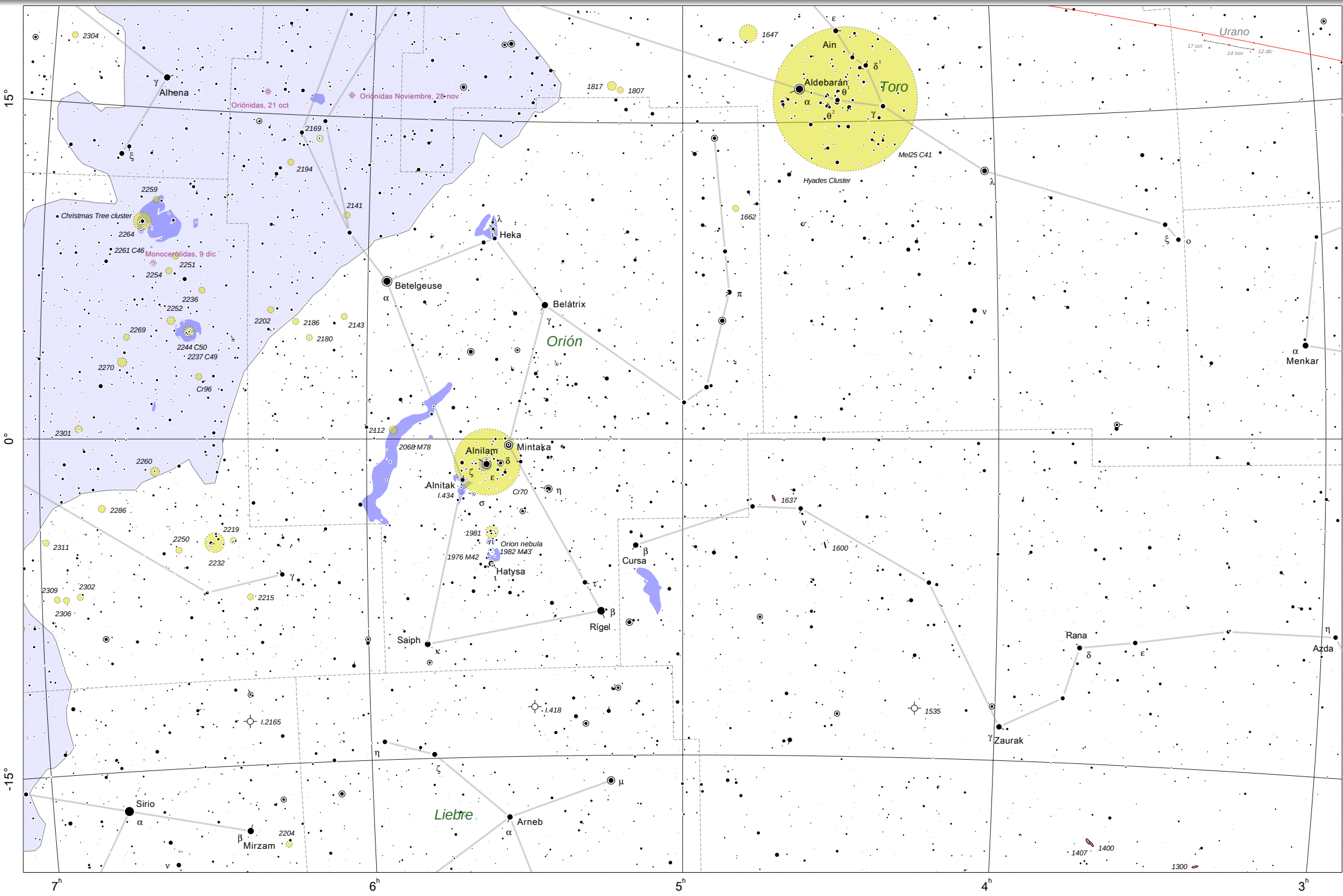
Carta 11, 30º alrededor de 5.0h, 0.0º (Orión, Erídano, Toro, Liebre)
