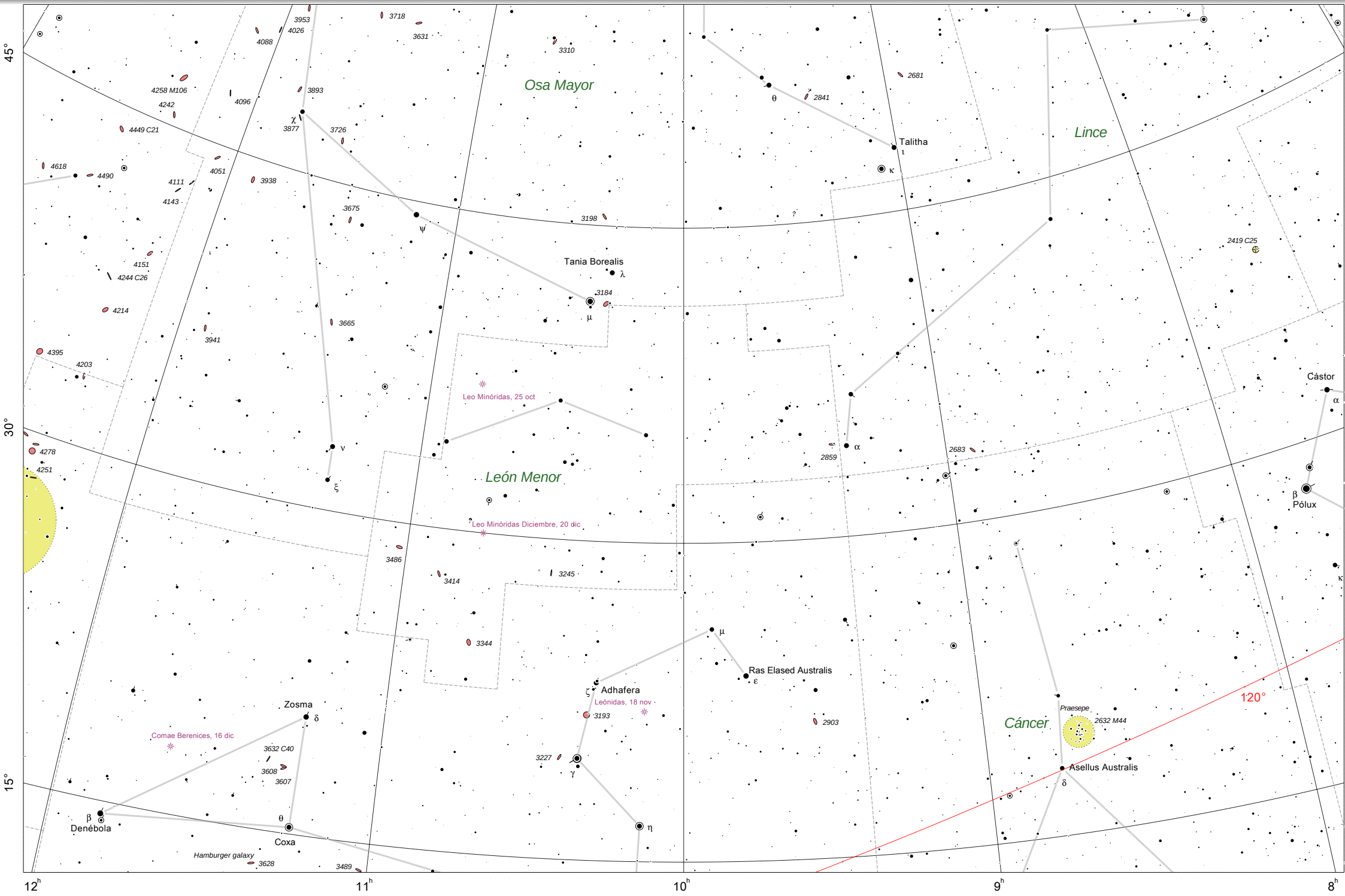
Carta 6, 30º alrededor de 10.0h, 35.0º (León Menor, Osa Mayor, Lince, Cáncer)
