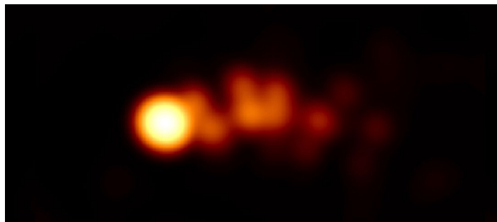
Imagen del blázar 1803+784 a una frecuencia de 7 GHz obtenida con interferometría de muy largas líneas de base (VLBI) en la que participó el radiotelescopio de 13m del Observatorio de Yebes.
