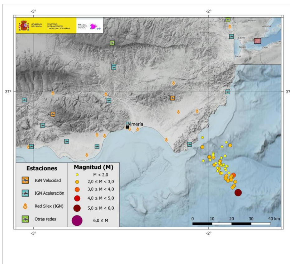
Figura 5. Mapa de estaciones sísmicas del IGN y otras instituciones más próximas a la zona epicentral que intervienen en la monitorización y cálculo de la actividad sísmica en tiempo real. Se incluyen los terremotos localizados en la zona desde el 14/07/2025 hasta la fecha.
