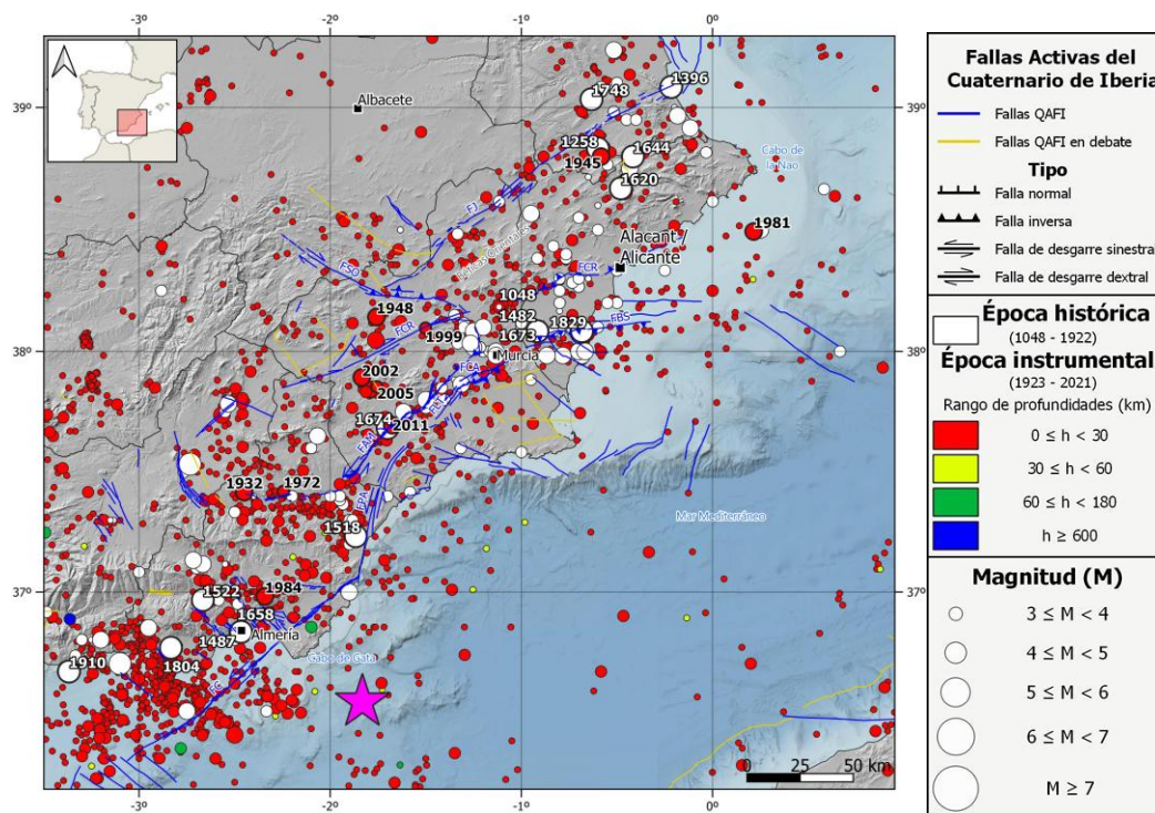
Figura 4. Marco sismotectónico de la zona y epicentro del terremoto principal de Mw 5,3 del 14/07/2025. La información sísmica proviene de la base de datos del Instituto Geográfico Nacional. Principales fallas activas durante el Cuaternario extraídas de la base de datos QAFI (IGME, 2022).
