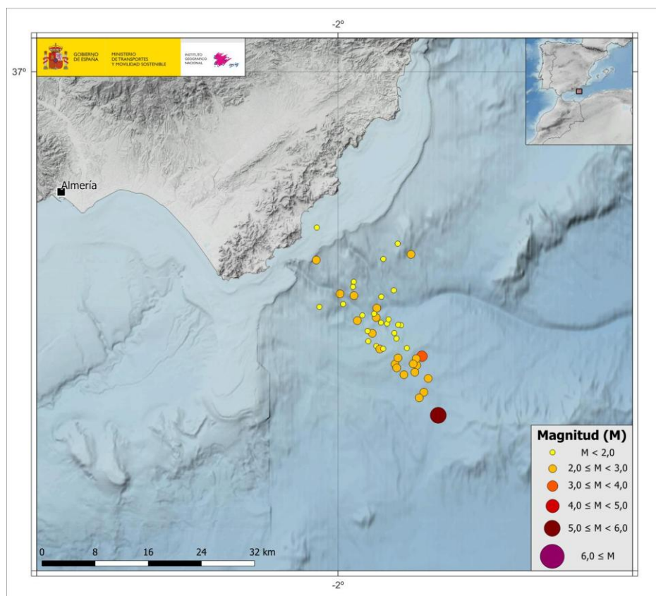
Figura 1. Mapa de sismicidad localizada en la zona epicentral desde el 14/07/2025 hasta la fecha.
