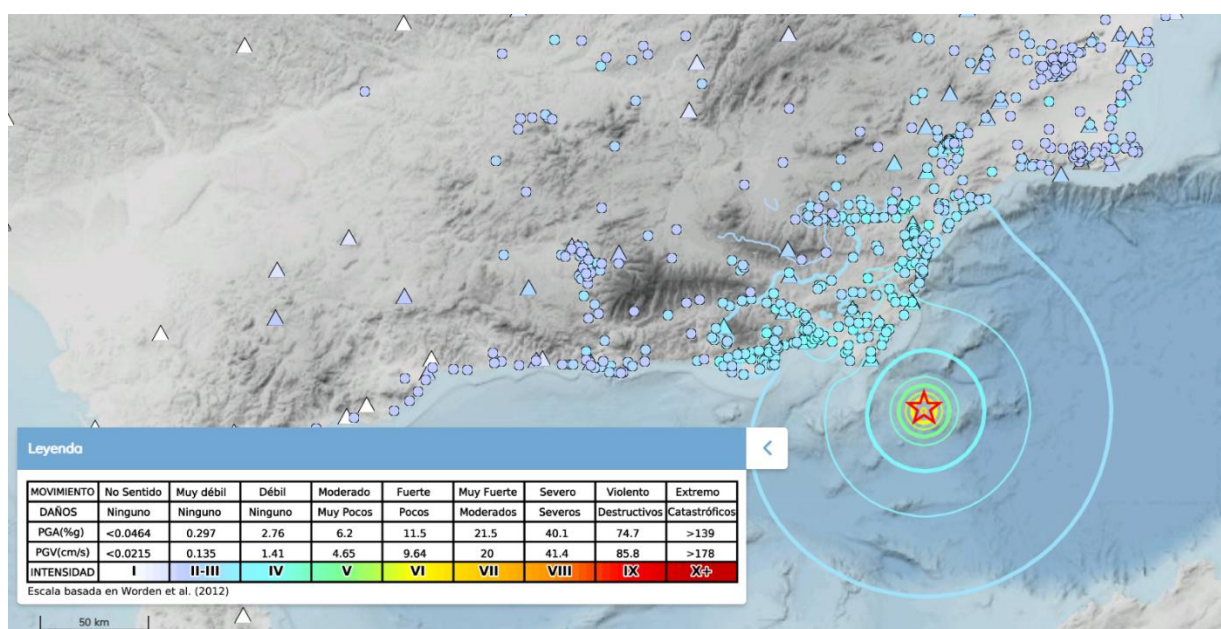
Figura 6. Mapa de isosistas de intensidad estimada a partir de datos puntuales de intensidad y datos de las estaciones sísmicas en el área regional del terremoto de Mw 5,3 del 14/07/2025. La leyenda inferior muestra las equivalencias utilizadas entre los parámetros usados para representar el movimiento del suelo.
