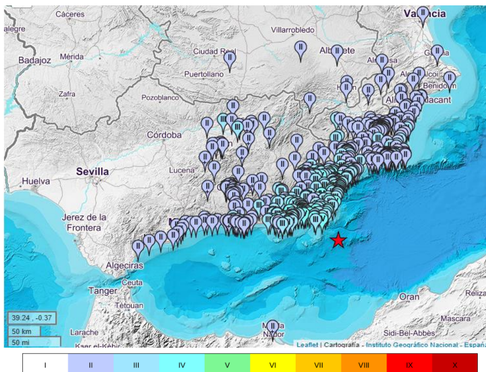
Figura 2. Intensidades registradas en España debidas al terremoto 14/07/2025 05:13:27 (UTC) ocurrido en la costa de Almería de Mw 5,3.
