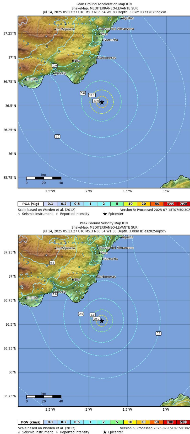
Figura 7. Shakemap de valores de PGA y PGV del terremoto de Mw 5,3 del 14/07/2025. La leyenda inferior muestra las equivalencias utilizadas entre los parámetros usados para representar el movimiento del suelo.
