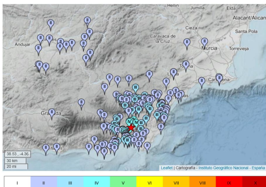
Figura 3. Intensidades registradas en España debidas al terremoto 15/02/2026 00:55:23 (UTC) ocurrido en Tabernas (Almería) de Mw 4,2.
