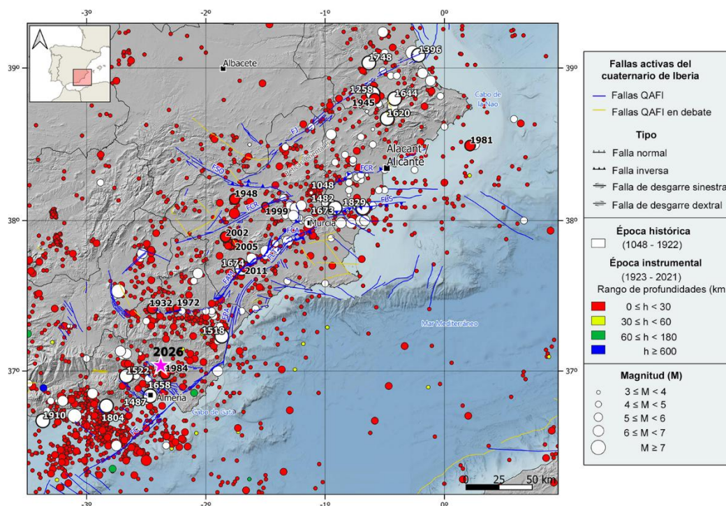
Figura 4. Marco sismotectónico de la zona y epicentro del terremoto principal de Mw 4,2 del 15/02/2026 (estrella negra). La información sísmica proviene de la base de datos del Instituto Geográfico Nacional. Principales fallas activas durante el Cuaternario extraídas de la base de datos QAFI (IGME, 2022).
