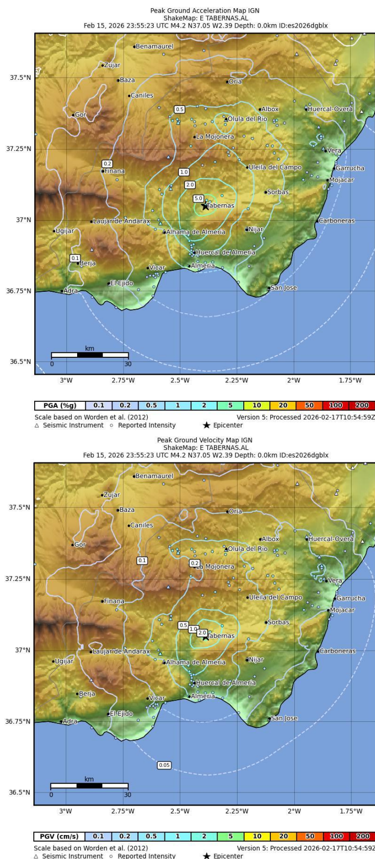
Figura 7 (continuación). Shakemap de valores de PGA y PGV estimados del terremoto de Mw 4,2 del 15/02/2026. La leyenda inferior muestra las equivalencias utilizadas entre los parámetros usados para representar el movimiento del suelo.
