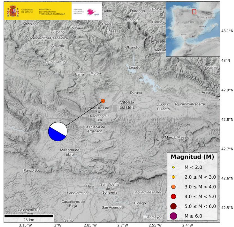
Figura 2. Mecanismo focal del terremoto principal de M_w 3,8 del 07/12/2025.
