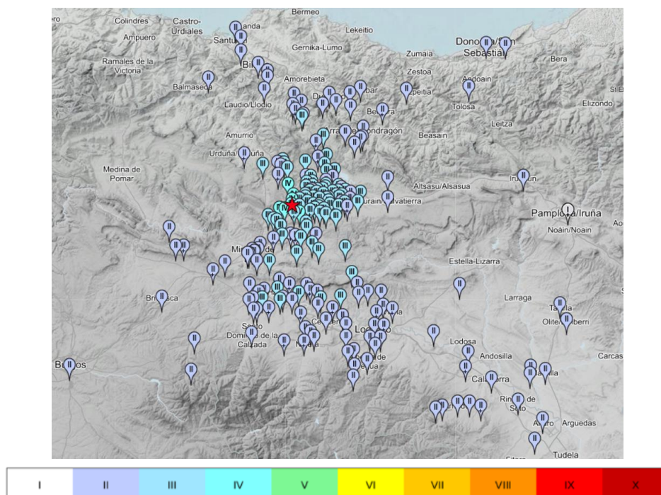
Figura 1. Intensidades registradas en España debidas al terremoto 07/12/2025 23:10:23 (UTC) ocurrido en la provincia de Vitoria-Gastéiz de Mw 3,8.
