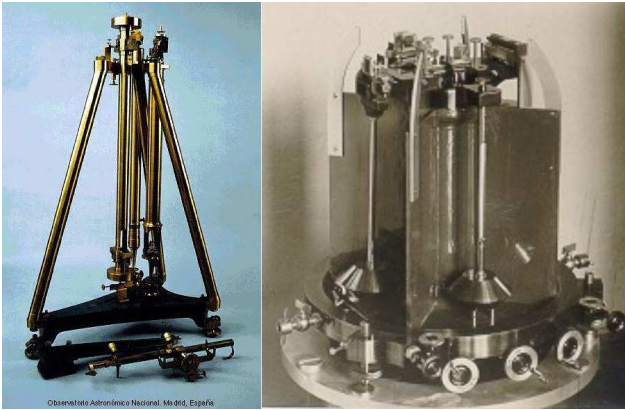
Figura 2: Péndulo de absolutas de Repsold (colección del OAN) y péndulo de relativas de Von Sterneck.
