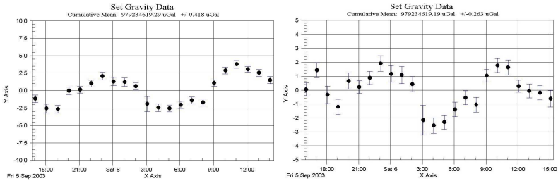
Figura 5: Observatorio IRAM de Pico Veleta (2850 m sobre el nivel del mar): antes y después de la corrección por carga oceánica.
