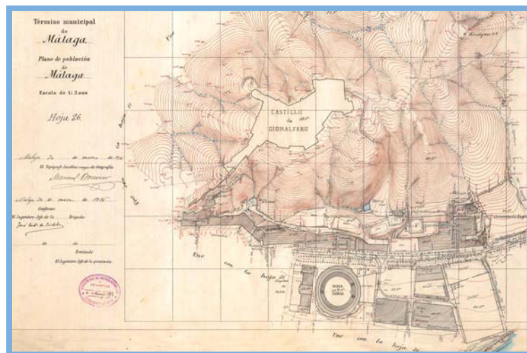
Fragmento del plano de población de Málaga, 1916, escala 1:2.000
