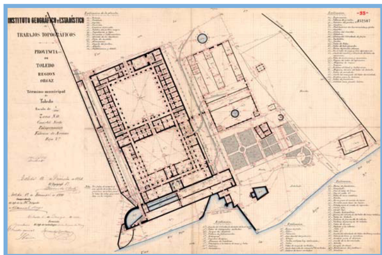
Plano de edificio de la Fábrica de Armas de Toledo, 1881, escala 1:500
